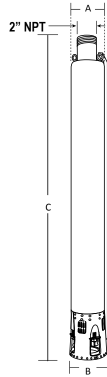
Acoplamiento NEMA 6"
